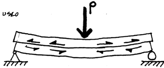
LONGITUDINAL SHEAR
